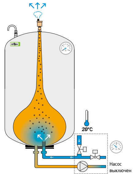
5. Заполнение Если уровень воды в емкости падает до критической отметки, то соответствующее количество воды будет заполнено в устройство через подпитку. Перед нагнетанием в систему вода дегазируется (вследствие понижения давления).
