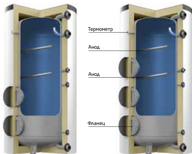
R2 - Два фланца AL 1500 - 3000/R2
