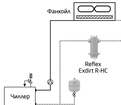
Exdirt "Сталь" - пример монтажа
