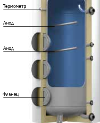
R3 - Три фланца AL 1500 - 3000/R3
