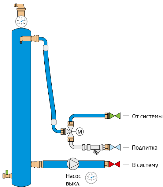
4. Ожидание Ожидание перед началом следующего цикла дегазации.
