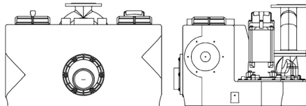
Рис. 3 Приёмный бак с местами подсоединения подводящих трубопроводов
