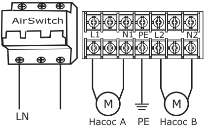
Рис. 12 Схема внешних подключений
