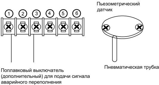
Рис. 13 Подключение реле уровня, порта диспетчеризации, внешней аварийной сигнализации
