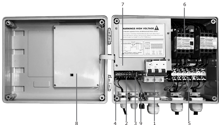
Рис. 11 Внешний вид шкафа управления
