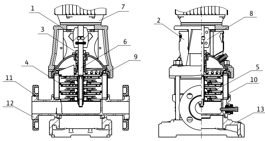
Рис. 1б. Насос в разрезе с указанием основных элементов (модель Helix VE 10-22)
