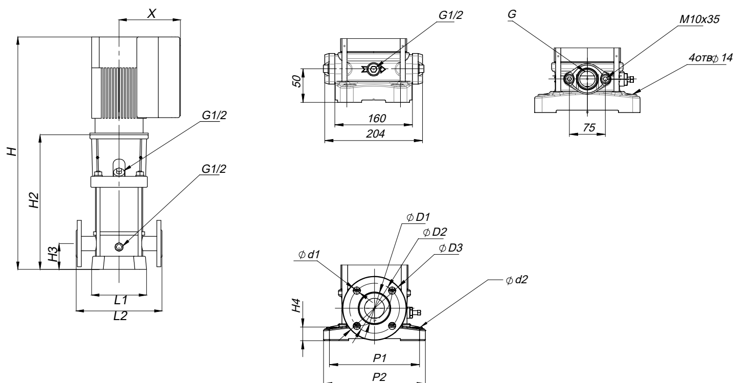
Рис. 4. Габаритный чертеж
