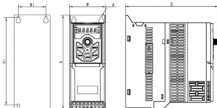
Типоразмер D1
